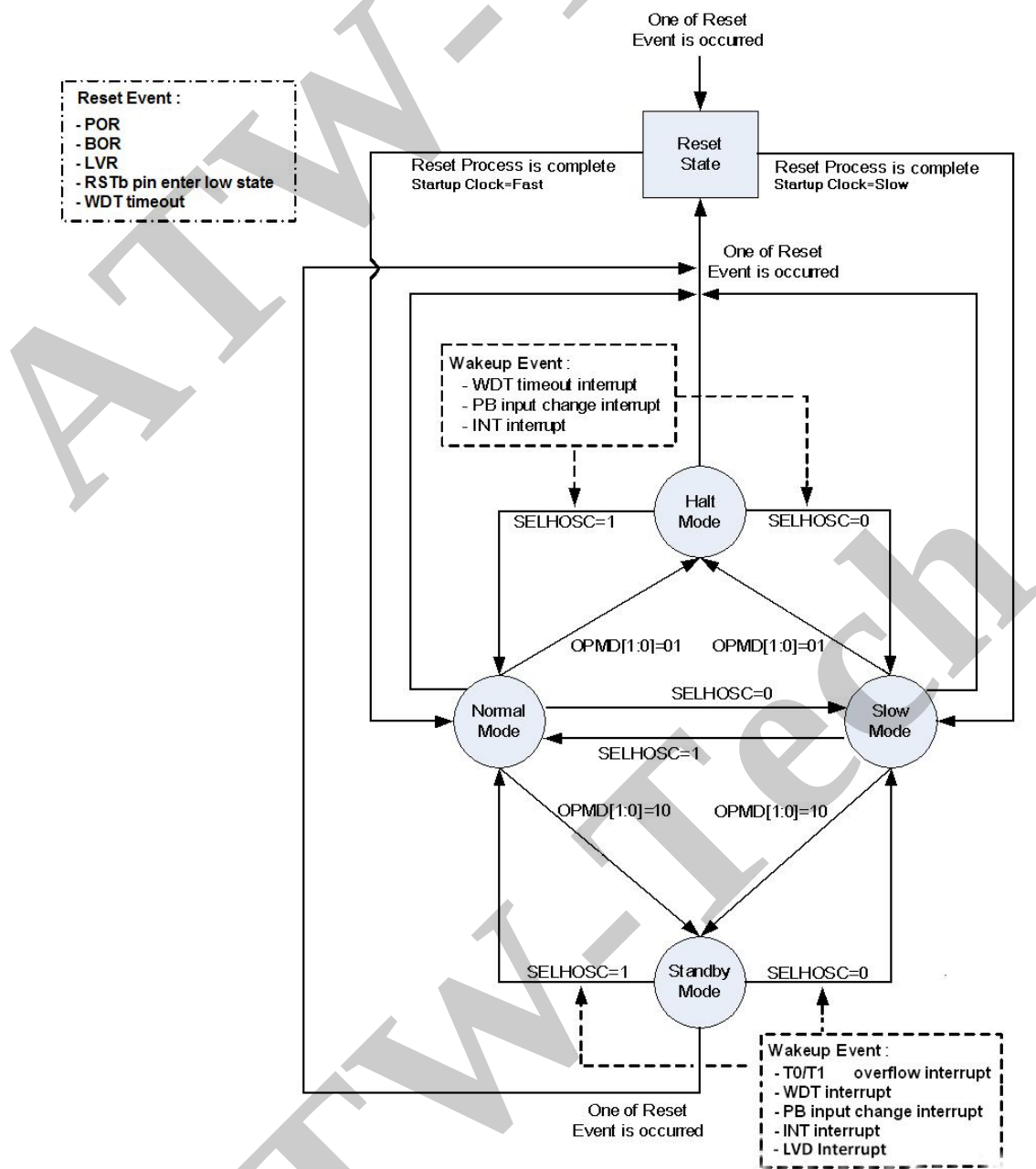
图 20 四种工作模式
