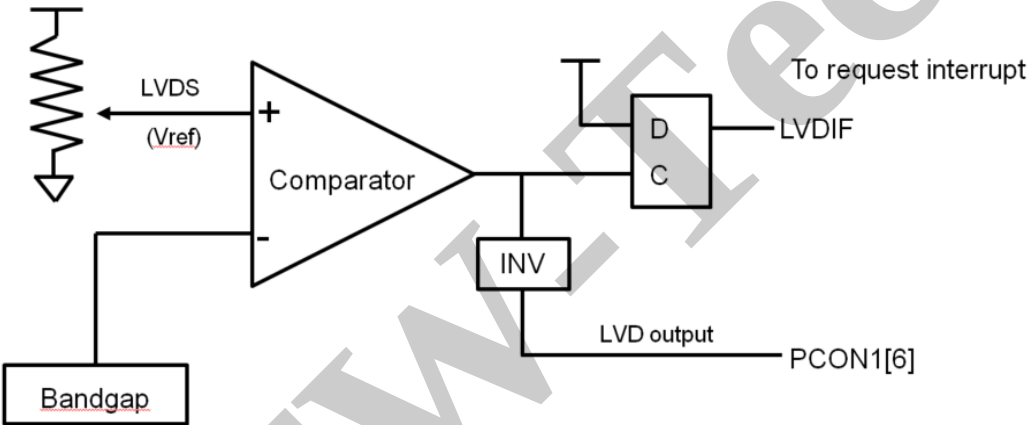
图 18 LVD结构框图
