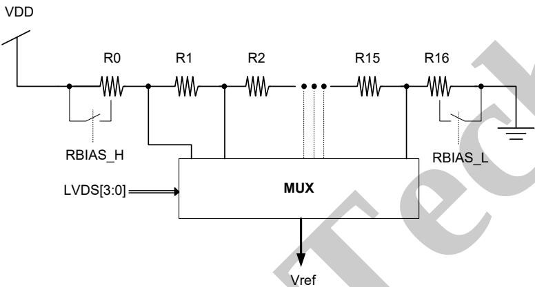
图 17 Vref硬件连接
