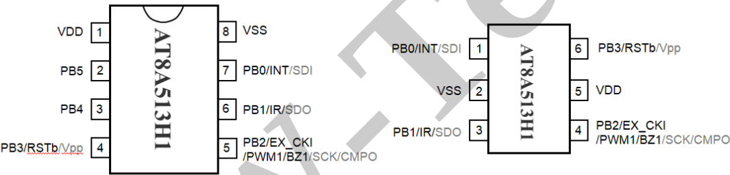
图 1 封装引脚图
