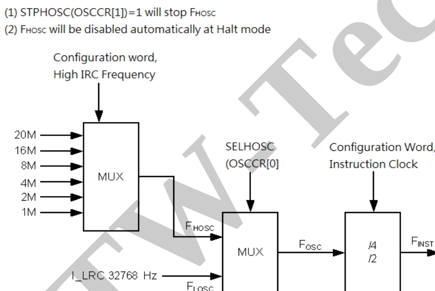
图 19 AT8A513H1 振荡配置结构图
