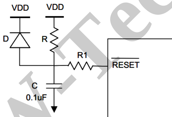
图 22 复位应用结构框图
