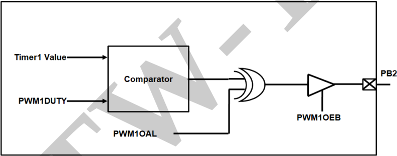
图 13 PWM1 结构框图
